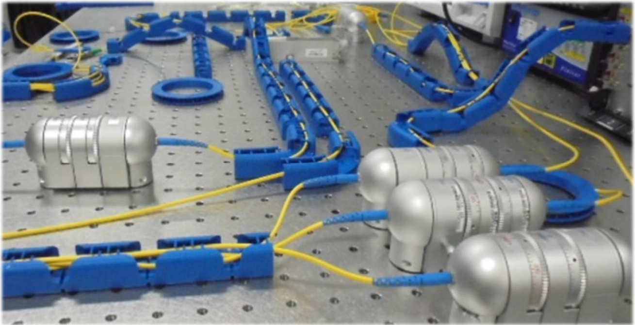
定盤上で光ファイバをアレンジ
